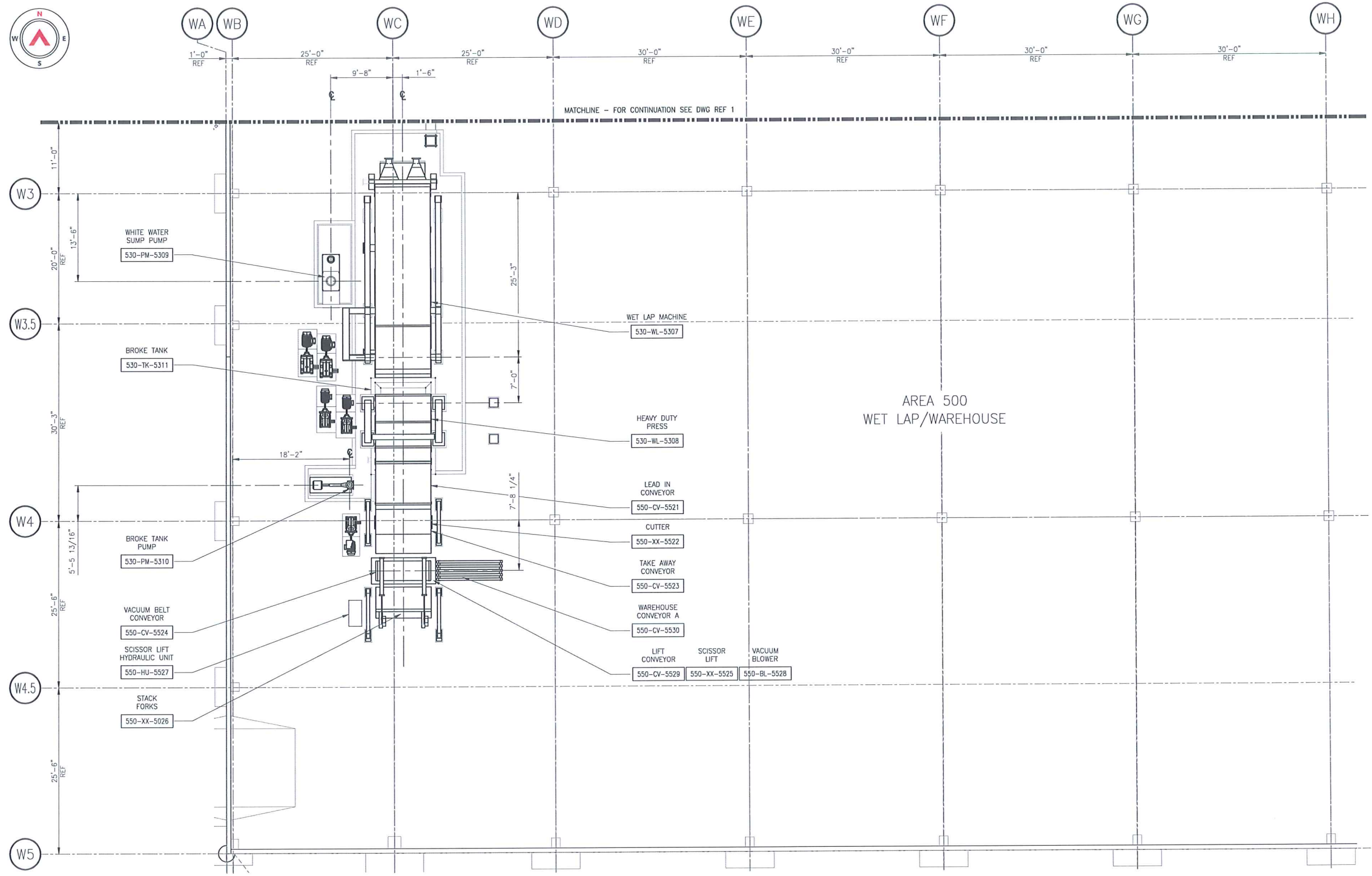
PLAN SCALE: 1/8"=1'-0"
